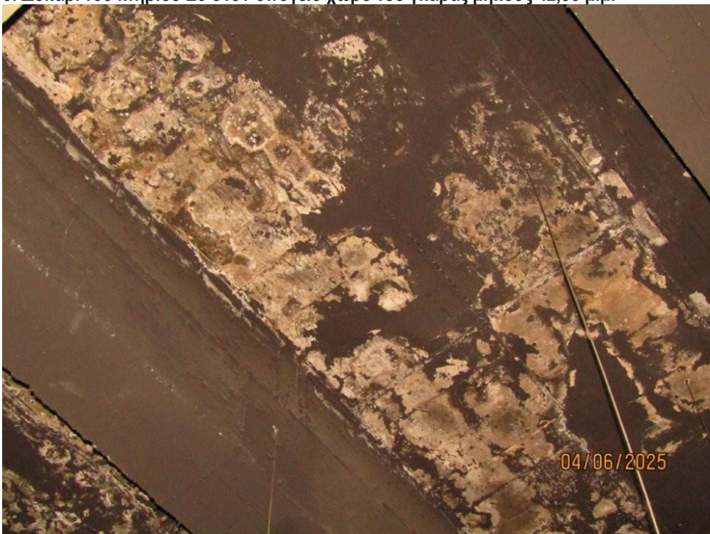
3. Δοκάρι του κτηρίου Ε5 στον υπόγειο χώρο του γκαράζ μήκους 42,38 μ.μ.
